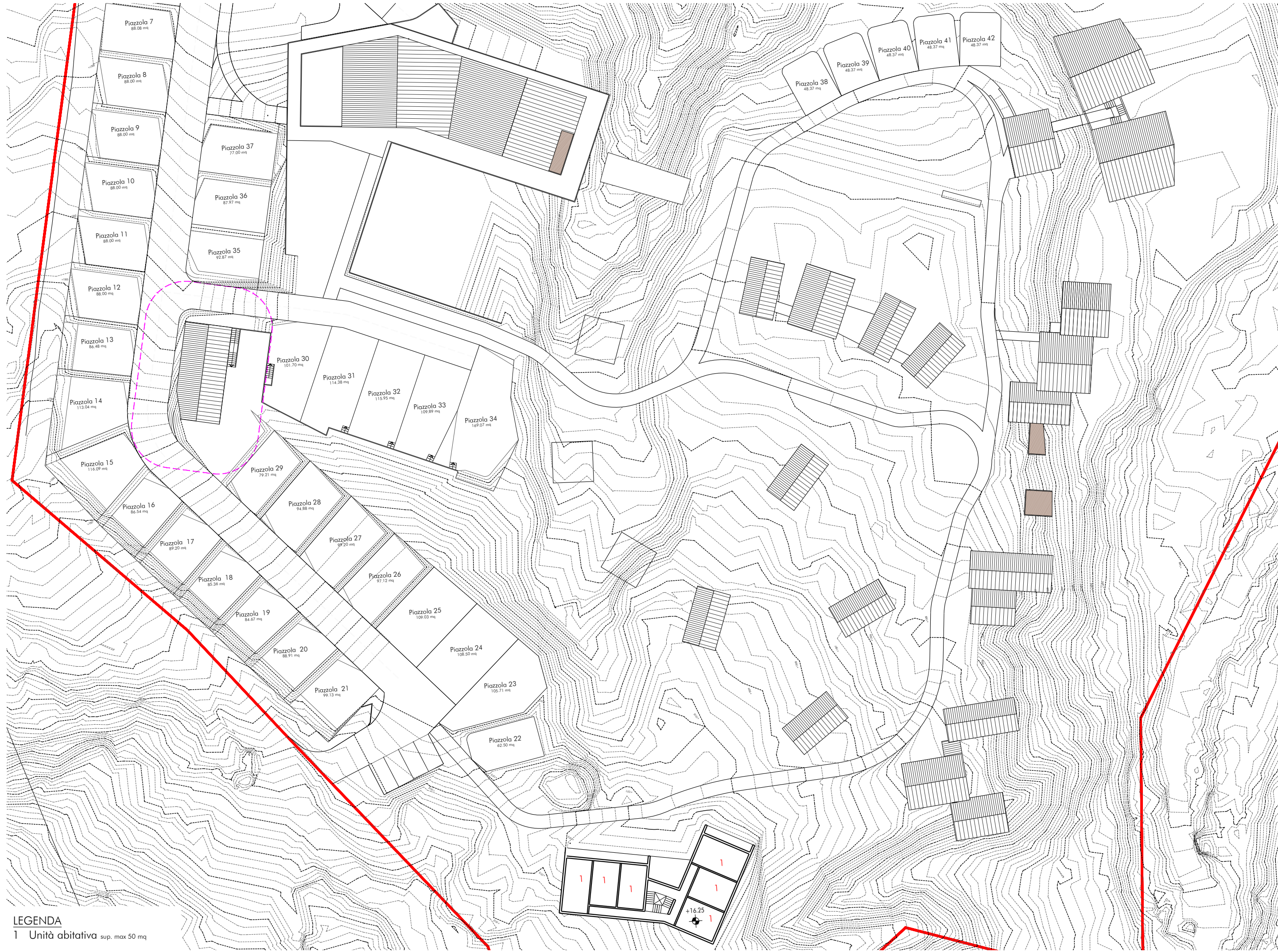
PIANTA QUOTA +1514.60/+16.25_ scala 1:500
